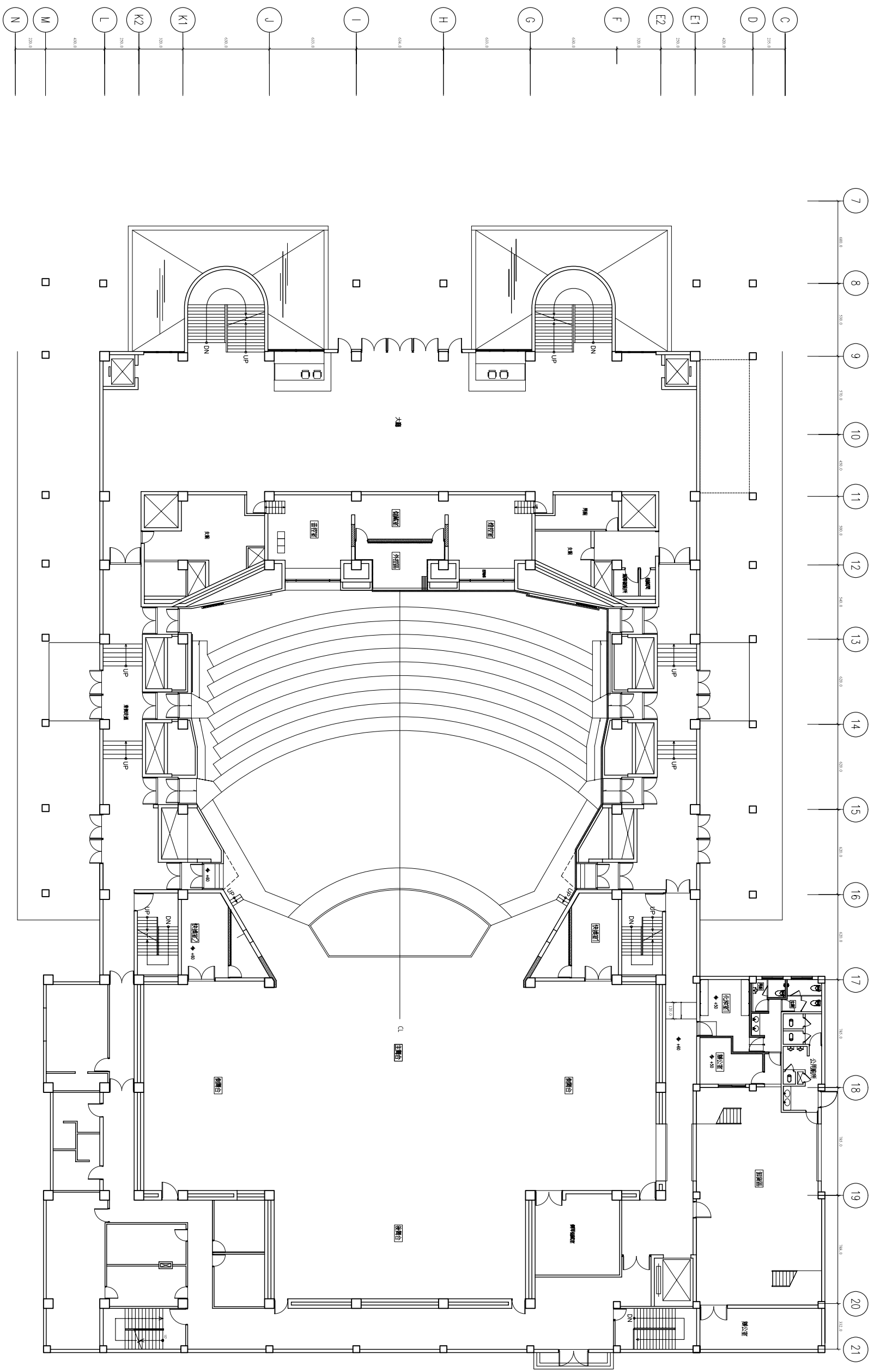
演藝廳一層平面圖 S:1/300
