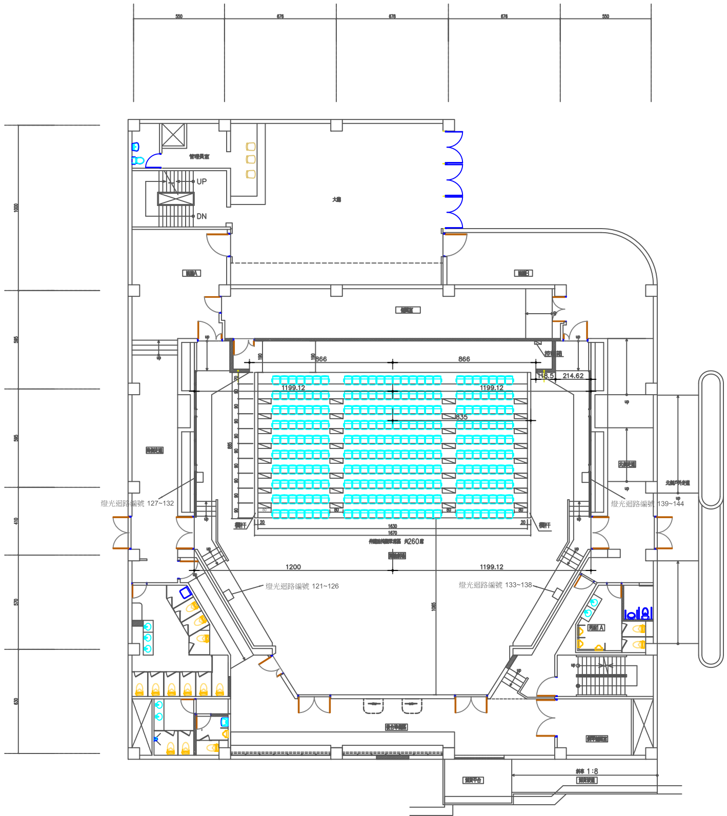
附件一：國際廳(原生劇場)一樓燈光迴路圖
