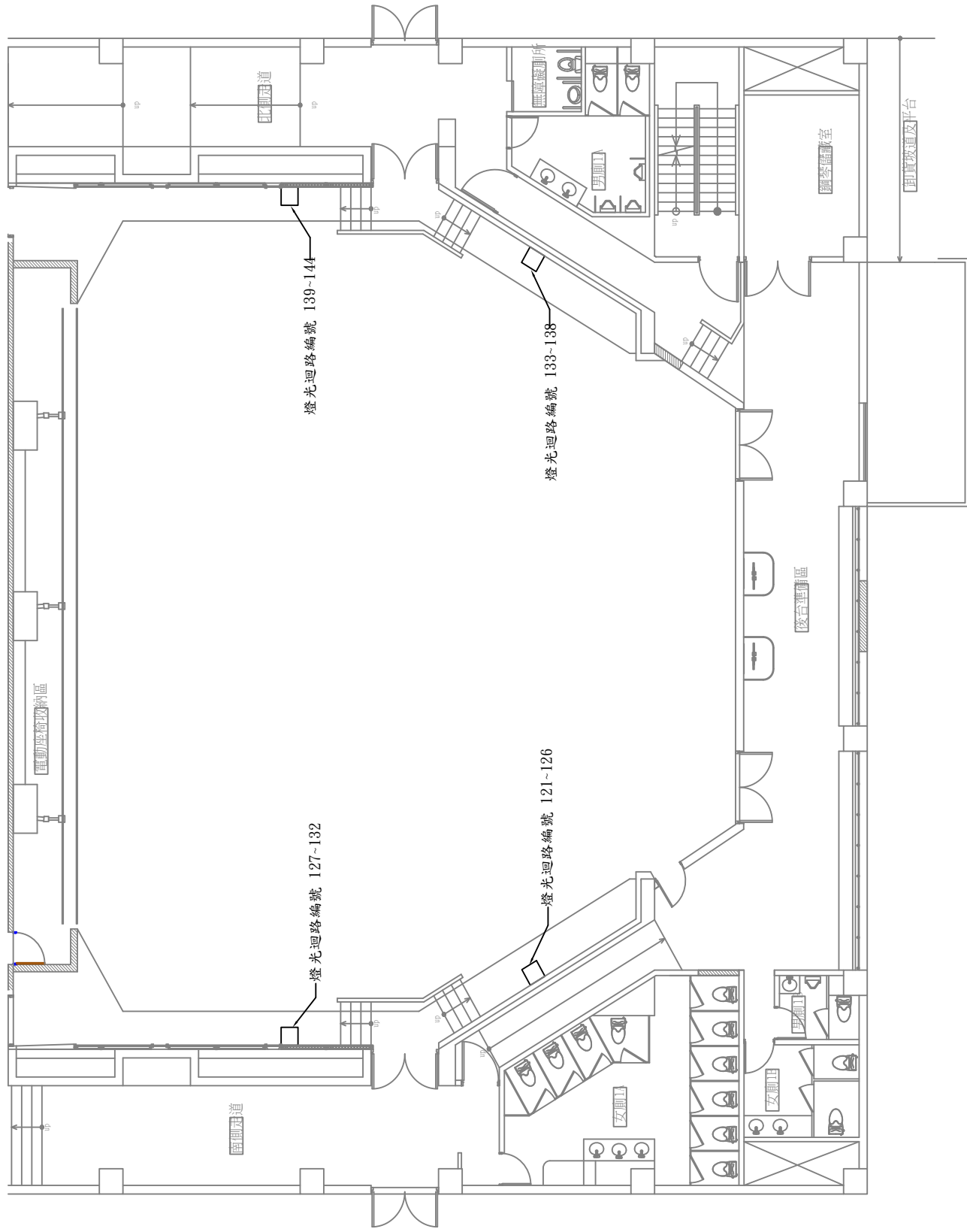
附件一：國際廳(原生劇場)一樓燈光迴路圖
